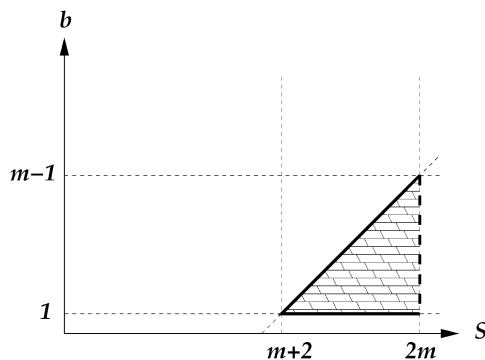
FIG. 1. Parameters (b, S) for a given m .
